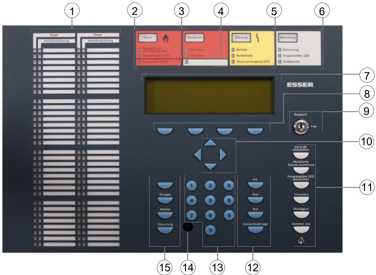
Abb. 1: Übersicht der Anzeige- und Bedienelemente
