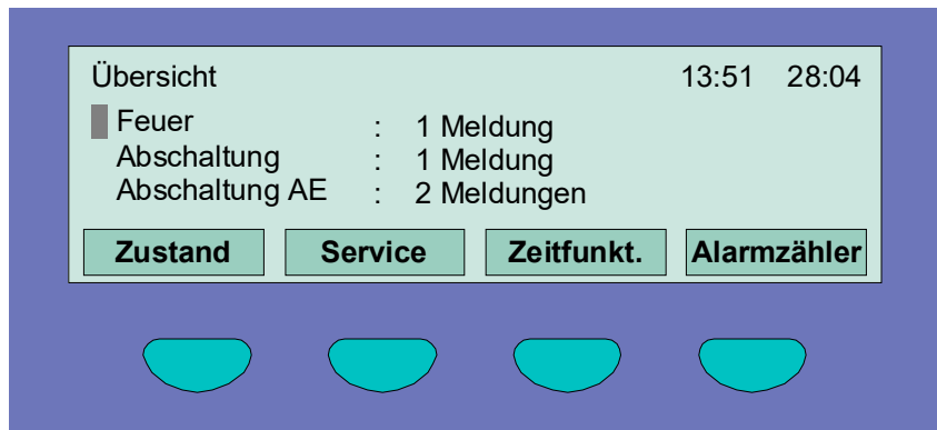
Abb. 41: Displayanzeige Übersicht
